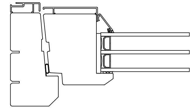
Vinklad profil insida - Vinklad glaslist utsida
