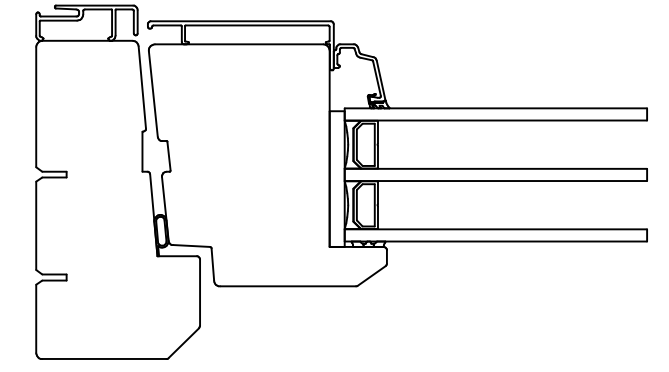
Vinklad profil insida - Rundad glaslist utsida
