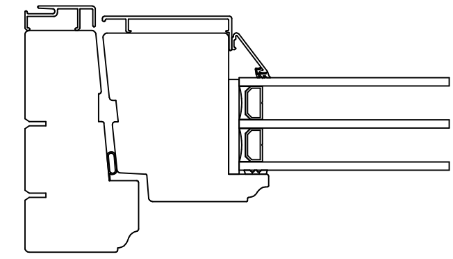
Rundad profil insida - Vinklad glaslist utsida
